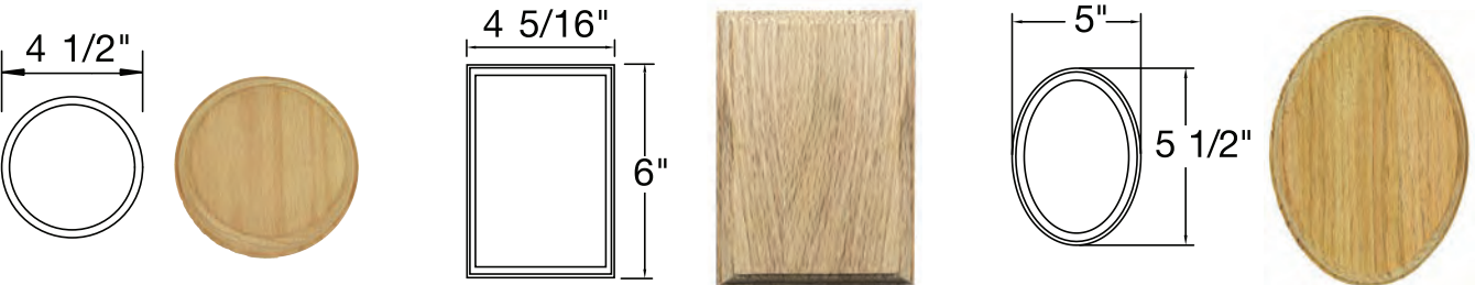
7317 • Round Rosette 7327 • Rectangle Rosette 7337 • Oval Rosette
